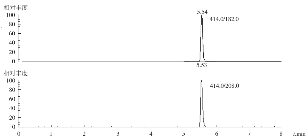
图 2 0.01 mg/L 草铵磷生物标准溶液色谱图
