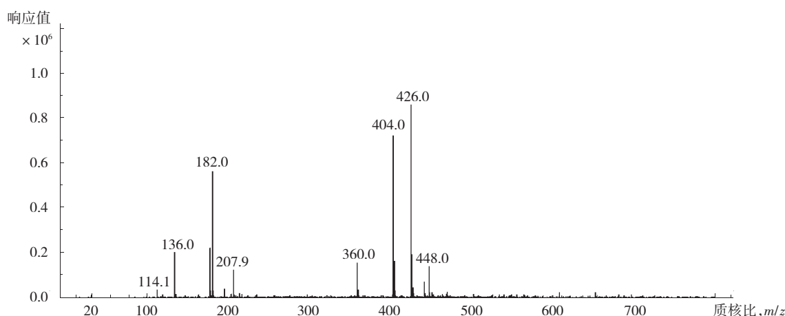
图 1 5 mg/L 草铵磷生物标准溶液的全扫描质谱图
